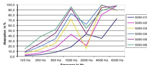
Luftschalabsorption DIN 52 215-63
